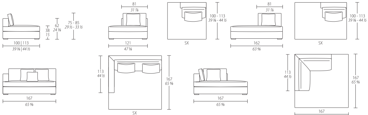
Isola Freestanding element Островной модуль
